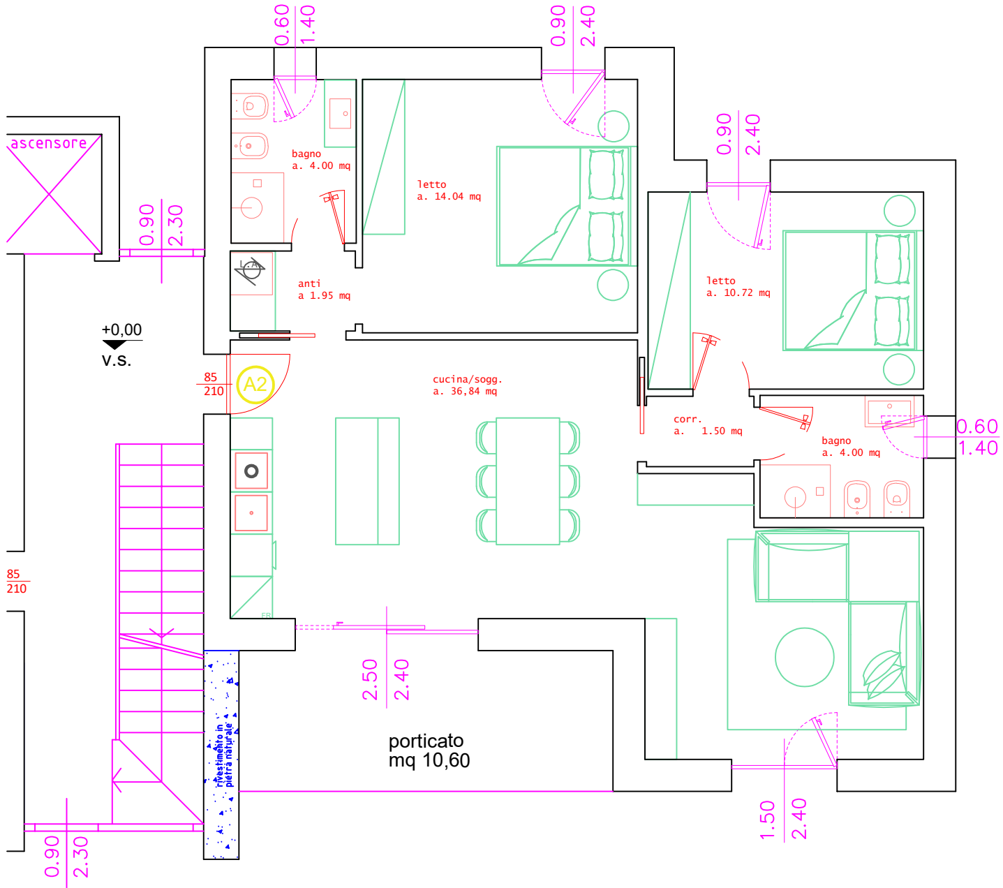
A2 - APPART. TRILOCALE PIANO TERRA
